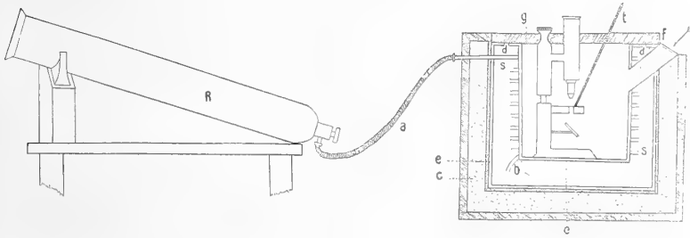
Fig. 1. — Schéma de l'appareil réfrigérant de Molisch, modifié de façon à produire le refroidissement à l'aide de l'acide carbonique liquide. — c , double enveloppe en bois remplie de sciure de bois ; ee , double enveloppe en cuivre nickelé ; dd , ouvertures de la boîte en cuivre ; g , couvercle en bois ; f , fenêtre ; ss , serpentin ; b , ouverture du serpentin à l'intérieur de la boîte en cuivre ; t , thermomètre, dont le réservoir s'appuie sur la platine du microscope, à côté de l'objectif ; a , raccord ; R , réservoir à acide carbonique liquide.
